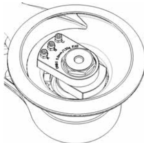
2. Maskinconfiguration til brug med Pad saver eller interface.
