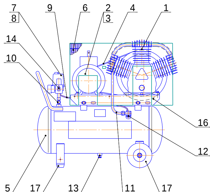
Рисунок 5 - Общий вид компрессора СБ4/С-50.ЛВ40
