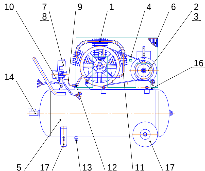
Рисунок 6 - Общий вид компрессора СБ4/С-100.ЛВ40
